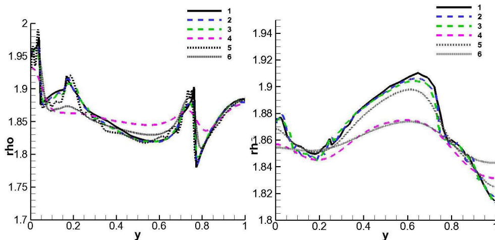
Рис.8. Плотность \rho вдоль линий 3 и 5, сетка h=1/400 , 1) эталонное решение, 2) VanLeer с числом Куранта Co=0.1 , 3) Minmod, 4) upwind, 5) КГД, \alpha=0.1 , Sc=0.0 , 6) КГД, \alpha=0.5 , Sc=0.0 .
